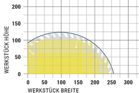
SCNITTDIAGRAMM
