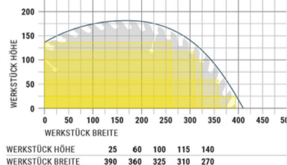
SCHNITTDIAGRAMM
